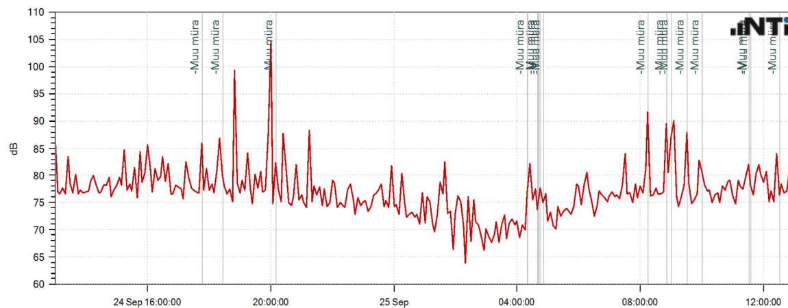
Graafik 2. Mõõtmispunktis MP2 mõõdetud maksimaalsed müratasemed L_{AFmax} . Hallide vertikaalidena on kujutatud muud mürasündmused.
