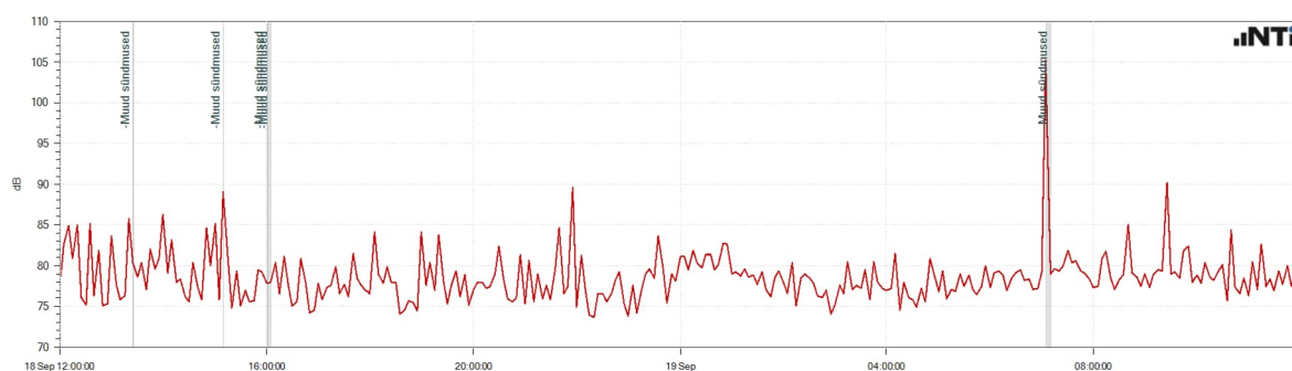
Graafik 1. Mõõtmispunktis MP1 mõõdetud maksimaalsed müratasemed L_{AFmax} . Hallide vertikaalidena on kujutatud muud mürasündmused.
