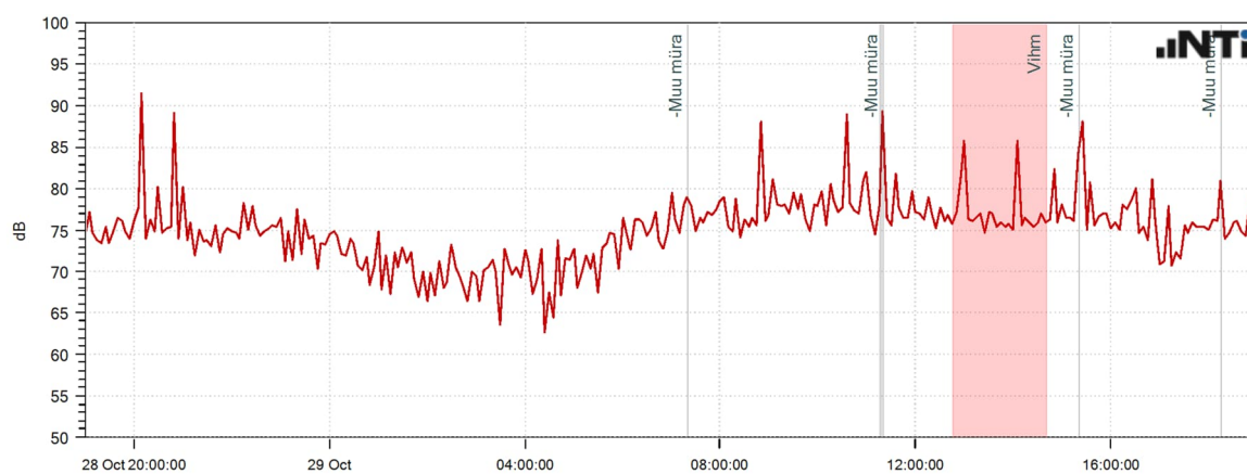
Graafik 1. Mõõtmispunktis MP1 mõõdetud maksimaalsed müratasemed L_{Amax} , 5min
