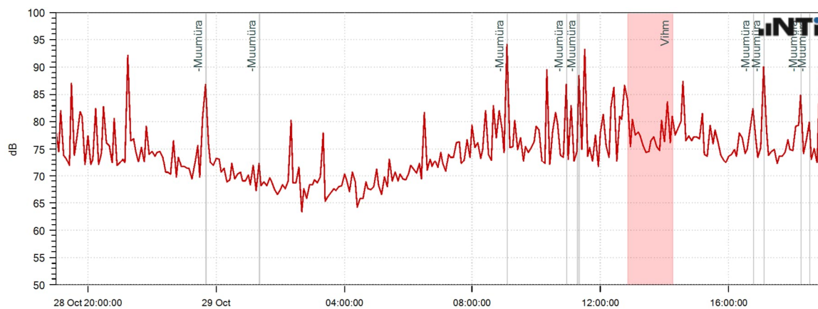
Graafik 2. Mõõtmispunktis MP2 mõõdetud maksimaalsed müratasemed L_{Amax} , 5min
