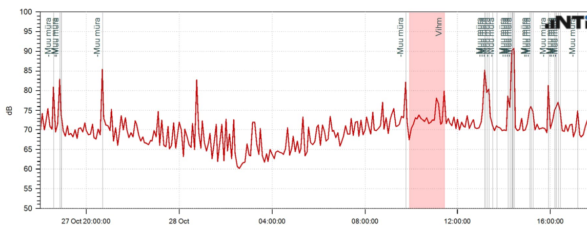
Graafik 1. Mõõtmispunktis MP1 mõõdetud maksimaalsed müratasemed L_{AFmax} , 5min
