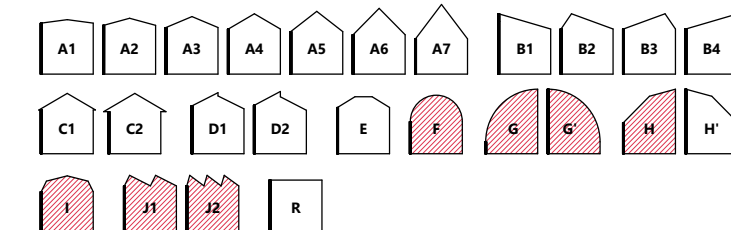
JOONIS 4.20 / UURITUD KATUSTE GEOMEETRIAD / ORIGINAALJOONIS [47, LK 1425]
