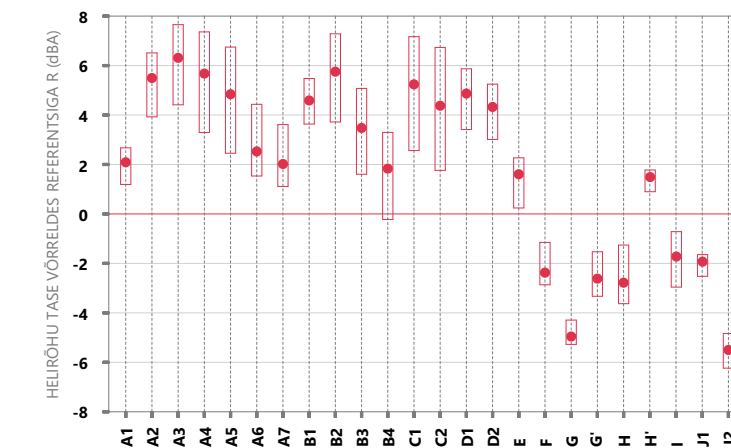
JOONIS 4.23 / AUTOLIKLUSEST PÕHIJATUD MÜRATASEMED UURITAVAL FASSAADIL VÕRRELDES REFERENTSOOLUKORRAGA R. / ORIGINAALJOONIS [47, LK 1428]
