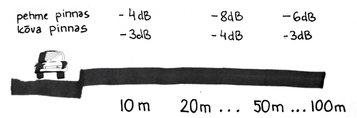
JOONIS 4.32 / HELITASEME VÄHENEMINE ERINEVATE PINNAKATETE KORRAL / ORIGINAAALJOONIS [63, LK 26]
