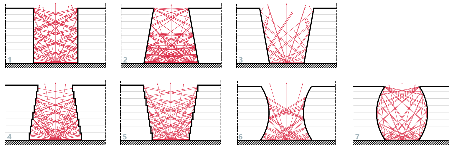
JOONIS 4.18 / HOONETE VERTIKAALSED VORMID / ORIGINAALJOONIS [43, LK 101]
