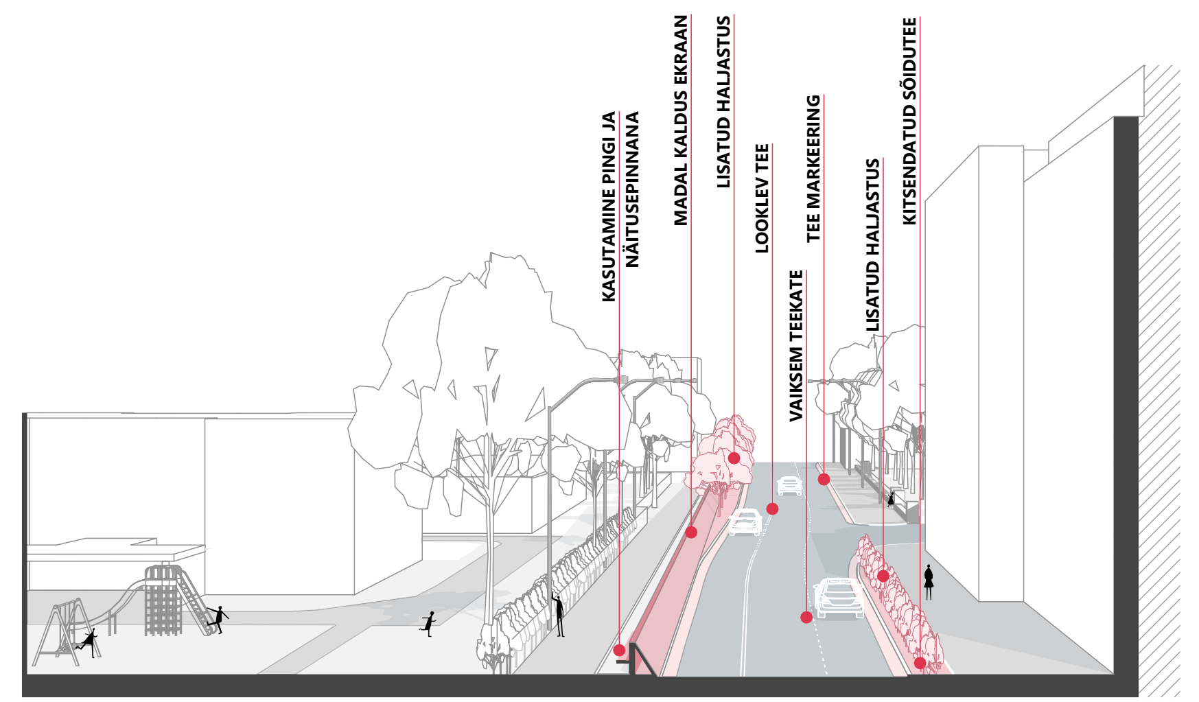
JUHKENTALI TÄNAVA LÕIGE
